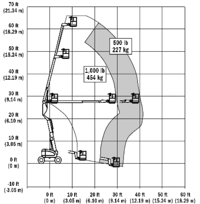
Diagrama de trabajo 600A
